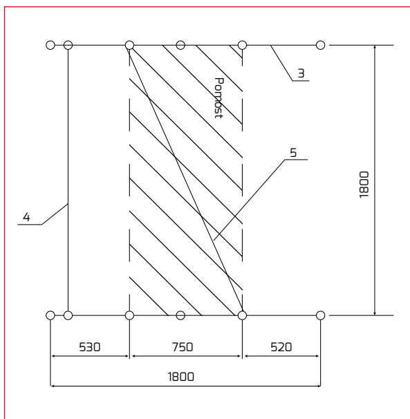
Ustawienie pomostu na belce jezdnej – symetryczne
