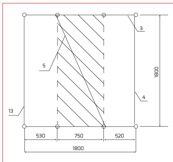
Ustawienie pomostu na belce jezdnej – symetryczne
