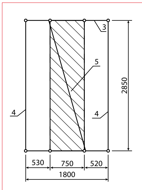
Ustawienie podstawy na belce jezdnej – symetryczne
