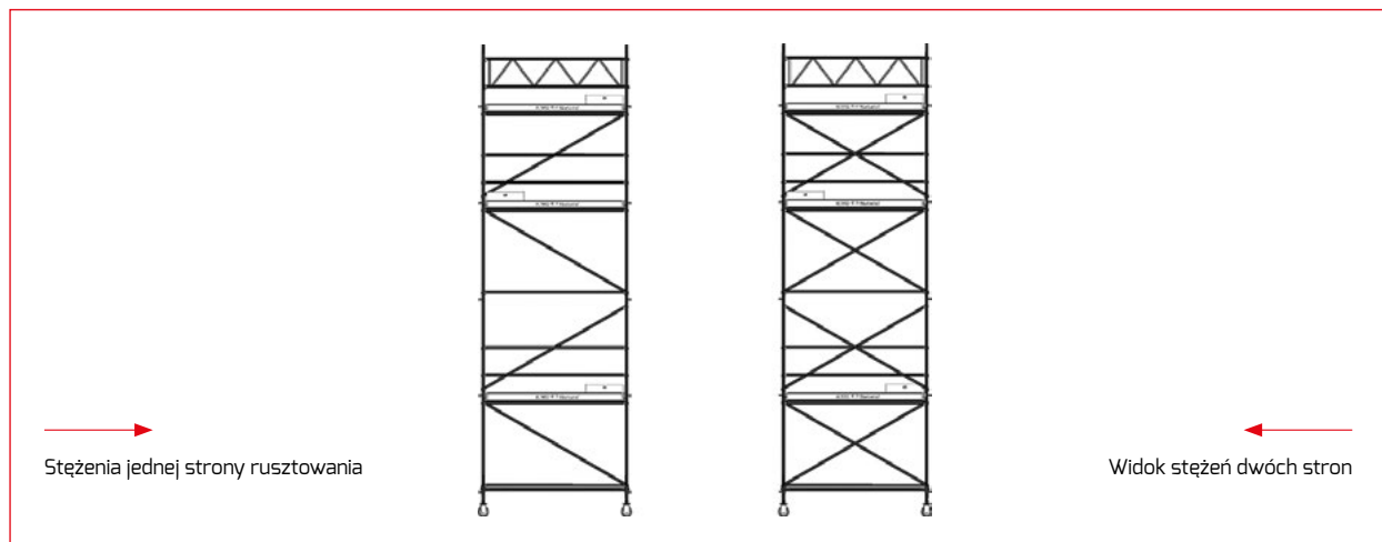
Rys. 1.8 Prawidłowo zamontowane stężenia
