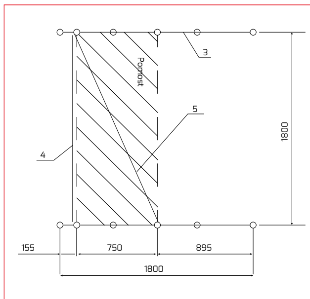
Ustawienie pomostu na belce jezdnej – niesymetryczne
