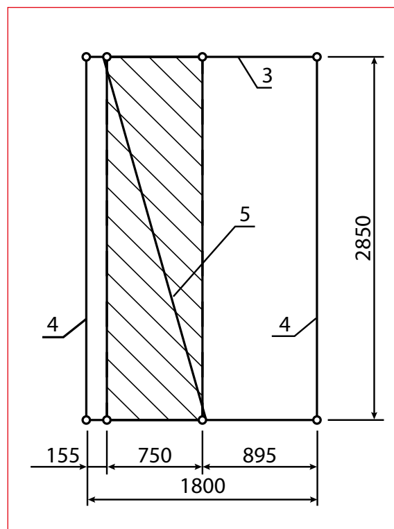
Ustawienie podstawy na belce jezdnej – niesymetryczne
