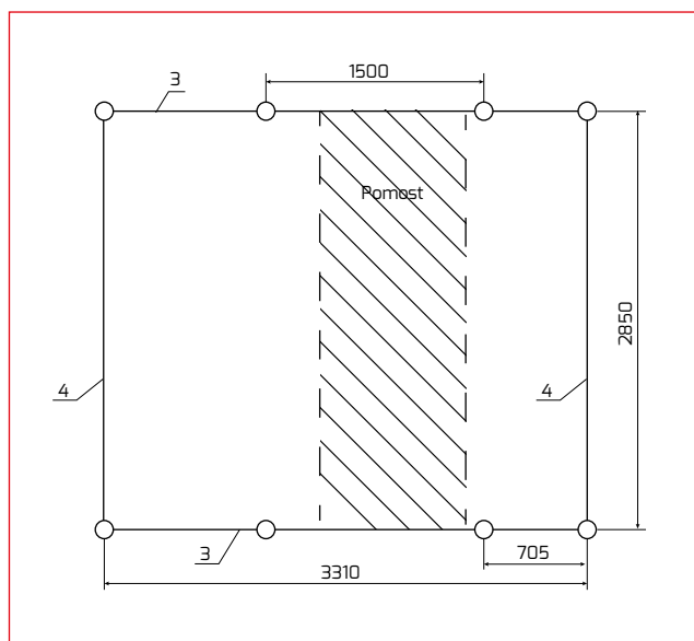
Ustawienie podstawy na belce jezdnej – niesymetryczne
