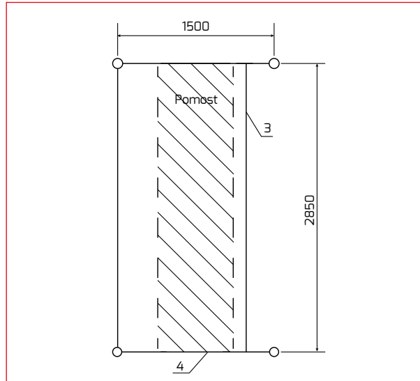
Ustawienie podstawy bez belki jezdnej
