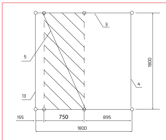
Ustawienie pomostu na belce jezdnej – niesymetryczne
