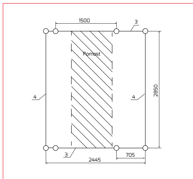
Ustawienie podstawy na belce jezdnej – symetryczne
